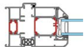
Jamb Detail
